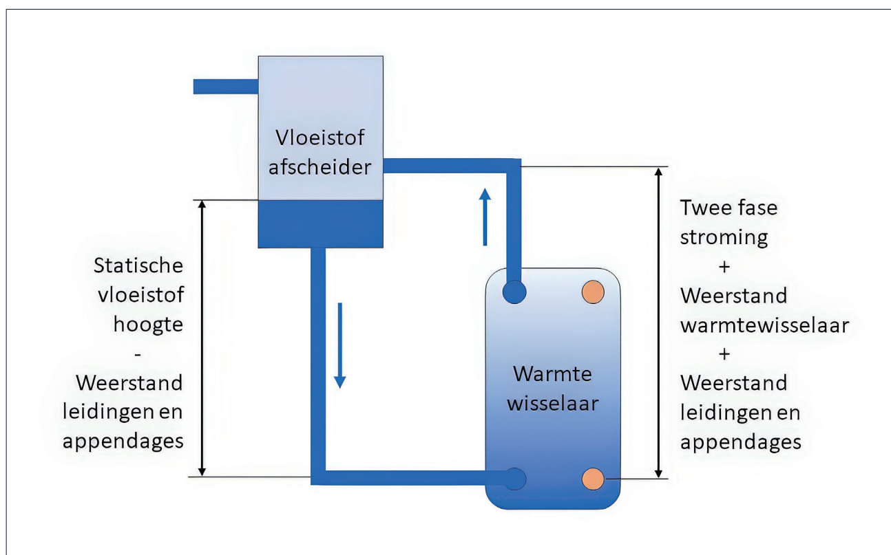
Fig. 3: De balans in een thermosyphon systeem.
