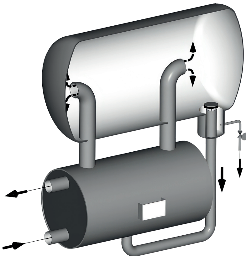
Fig. 1: Een thermosyphon verdamper met afscheider.
