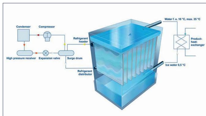
Fig. 4: Principe van een split tank (HTT-Buco).
