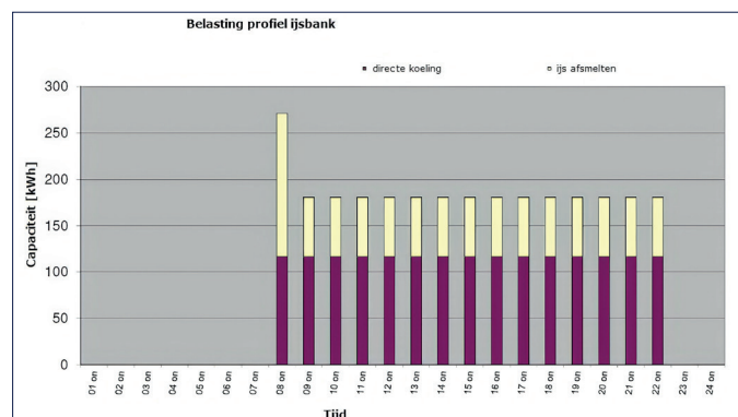
Fig. 3: Voorbeeld van een belastingprofiel van een ijsbank.
