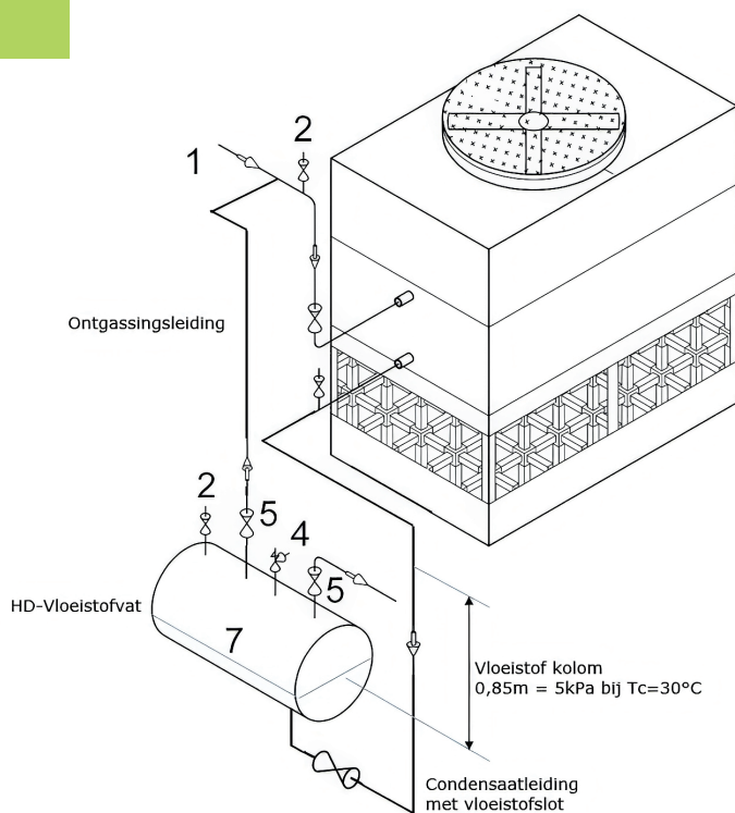
Fig. 2: Condensor aangesloten met vloeistofslot.
