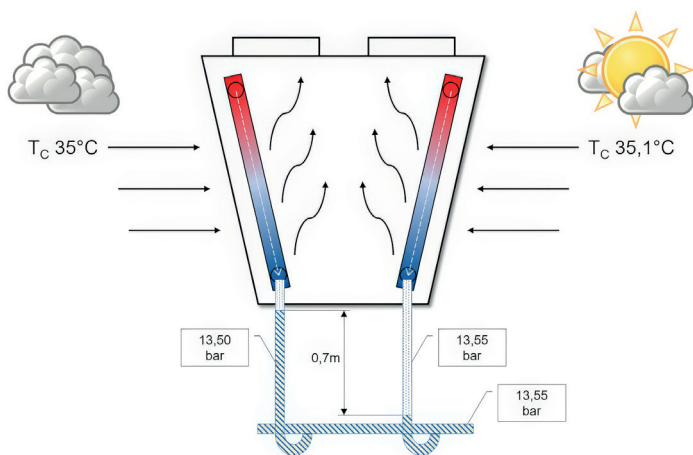
Fig. 3: Twee condensorcircuits op één vlotter.
