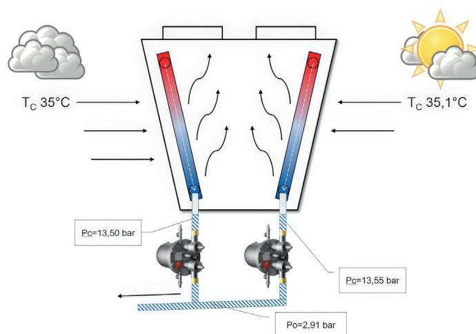
Fig. 4: Hogedrukvlotter per circuit.
