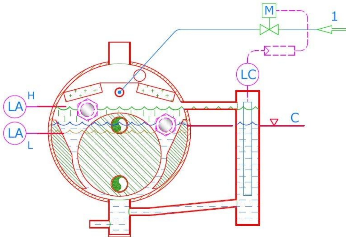
Afb 3. Badverdampster met ingebouwde afscheider.
